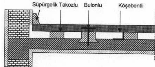
Şekil 1. Kadronların Döşemeye Bağlantısı
