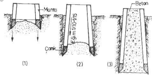
Şekil 1. Açık Keson Uygulama Aşamaları
