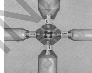
Resim 1. Uzay Çatı Sistem Elemanlarının Düğüm Noktası
