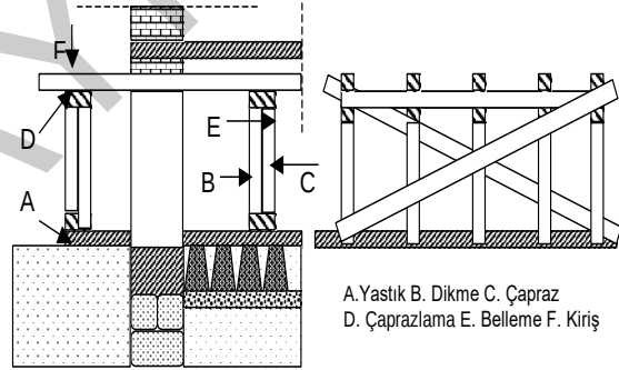
Şekil 1. Binanın Bir Kısımının Askıya Alınması
