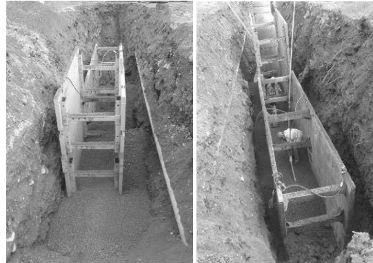
Resim 1. Basit Kanal İksa Uygulamaları
